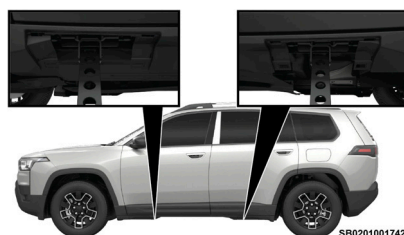
Puntos de levantamiento
