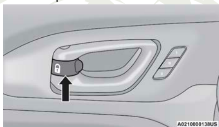
Seguros manuales de las puertas
