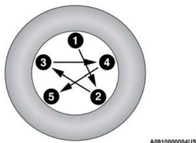
Patrón de apriete
