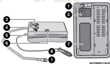
Componentes del kit de reparación
