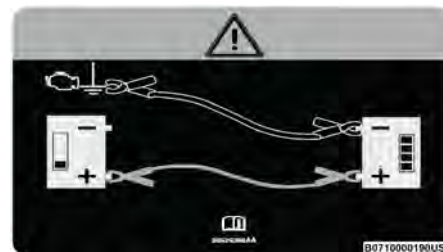
Procedimiento de arranque con cables pasacorriente
