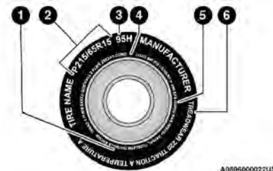
Marcado de la llanta
