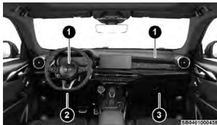
Ubicaciones de las bolsas de aire y protectores de rodilla (si así está equipado)
