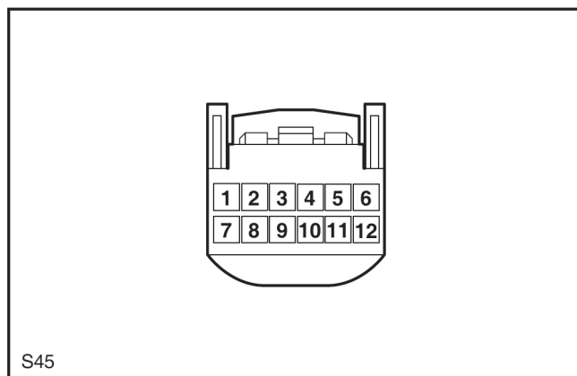
Interruptor del EPB
