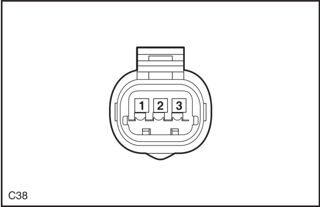
Motor de ajuste del faro derecho delantero
