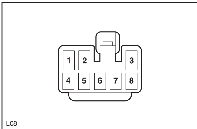
Luz de techo frontal
