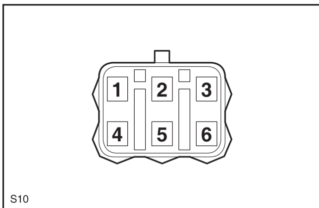
Luz izquierda trasera
