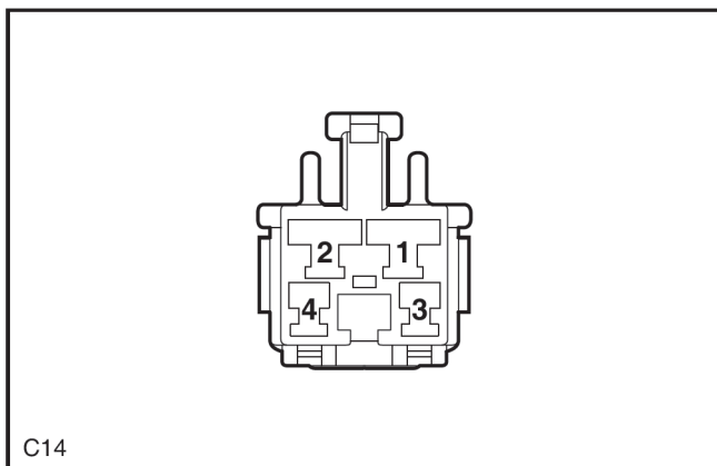
Interruptor de freno
