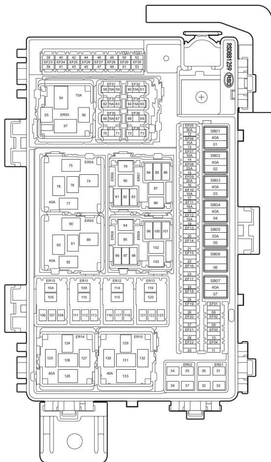
Caja de fusibles del compartimiento del motor
