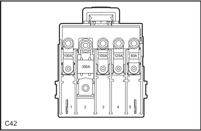
Caja de fusibles de la batería
