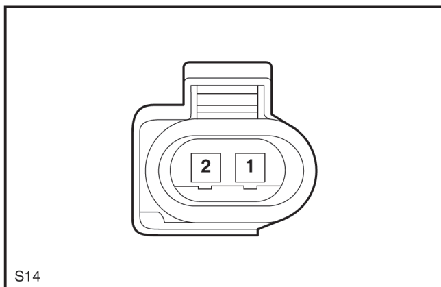
Motor izquierdo del freno de estacionamiento eléctrico
