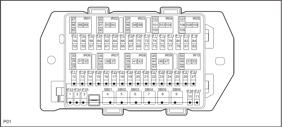
Caja de fusibles del tablero de instrumentos
