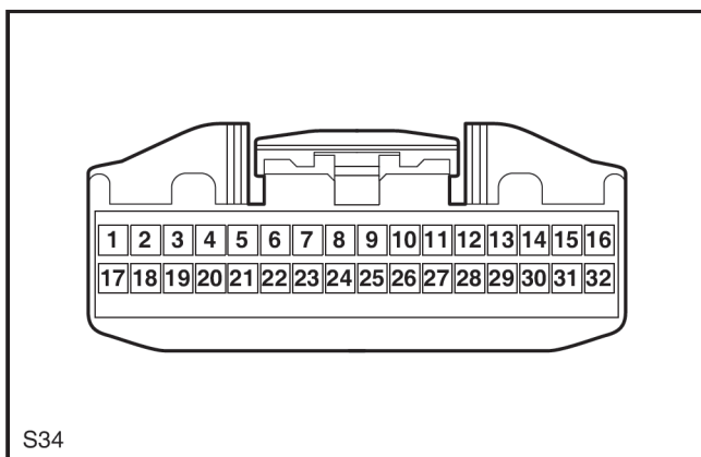
Control del radar de reversa
