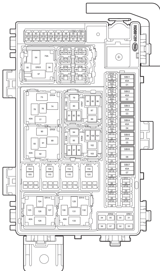
Caja de fusibles del tablero de instrumentos
