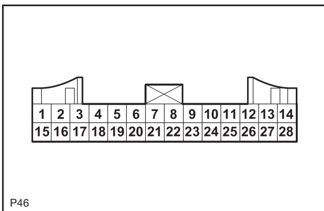
Módulo de interruptores izquierdo del tablero de instrumentos
