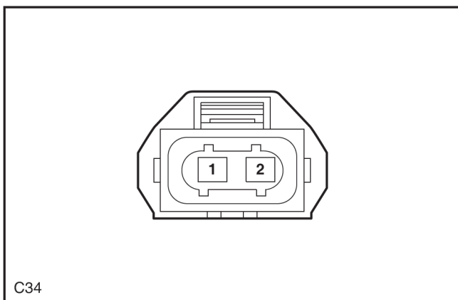
Luz de circulación diurna derecha delantera
