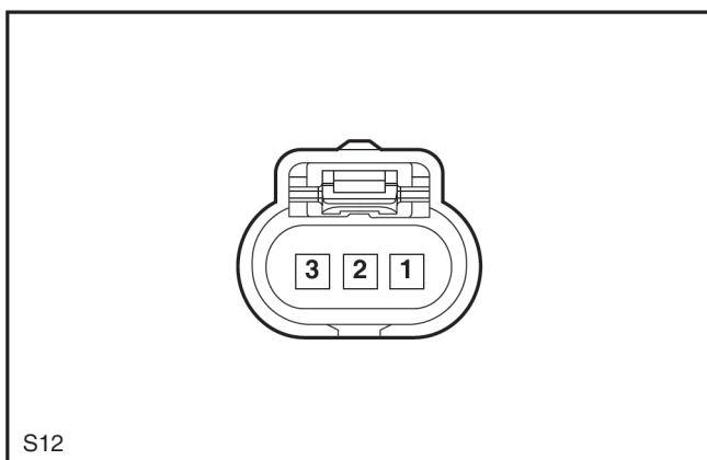
Sensor radar de reversa del centro izquierdo
