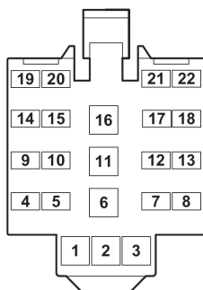
Arnés eléctrico del chasis hacia arnés eléctrico del piso A
