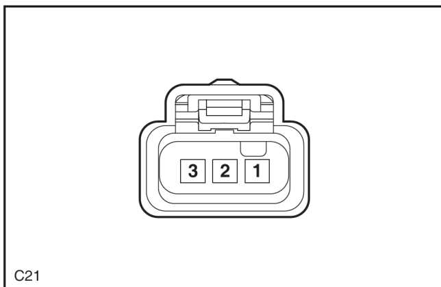
Sensor radar de la esquina izquierda delantera
