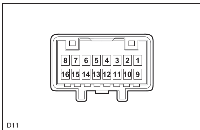
Espejo retrovisor derecho
