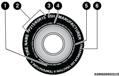
Marcado de la llanta
