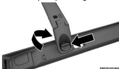
Instalación de las barras laterales
