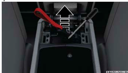
Liberador de la bisagra
