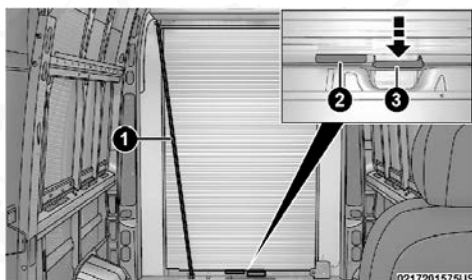
Operación interior de la puerta de cortina
