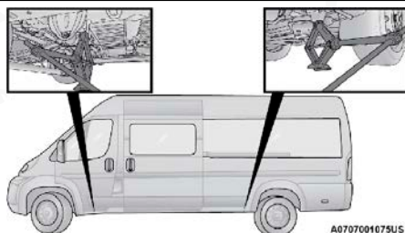
Posiciones de colocación del gato
