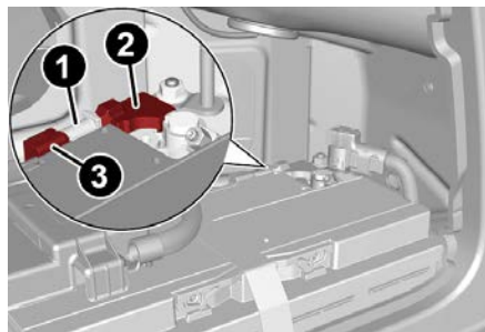
Suministro de energía a la batería
