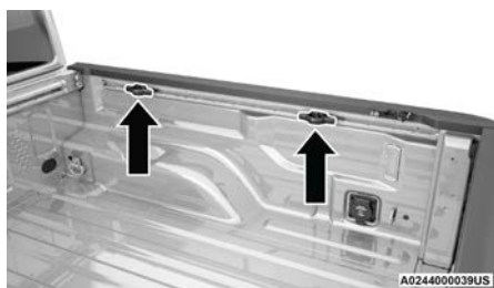
Ubicación de los anclajes en la batea
