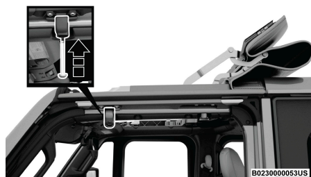
Coloque el tornillo del riel de la puerta delantera
