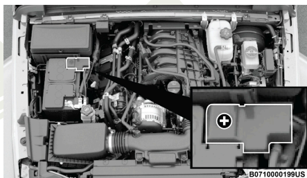
Poste positivo de la batería-Motor a gasolina
