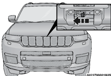
Localización del broche de seguridad
