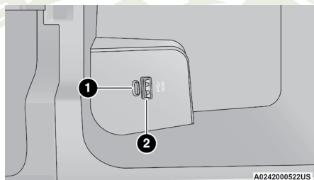
Puertos USB de carga en el compartimiento central trasero
