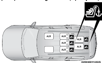
Ubicación de los retrectores de bloqueo automático (ALR) en vehículos de asientos 60/40 en la segunda fila (7 pasajeros)
