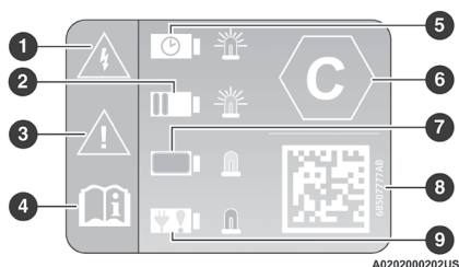
Etiqueta de advertencia de entrada de carga
