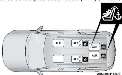
Ubicación de los retrectores de bloqueo automático (ALR) en vehículos de asientos tipo capitán en la segunda fila (6 pasajeros)
