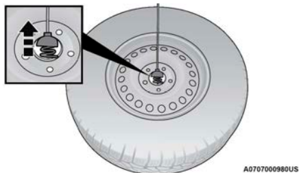
Librando el retenedor
