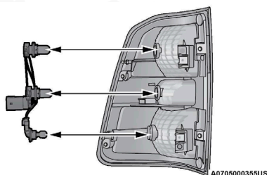
Árnés del conector de luces
