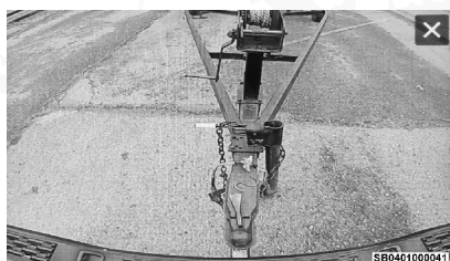
Acoplador del remolque ensamblado correctamente
