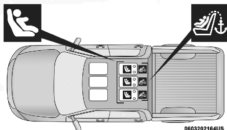
Ubicación de los anclajes LATCH en modelos Crew Cab® con asiento de banca dividida 60/40
