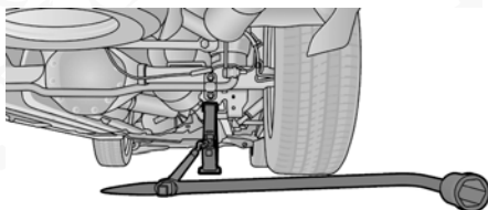
Punto de levantamiento trasero
