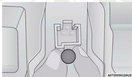
Retiro/instalación del foco
