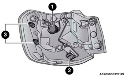
Parte trasera de la calavera
