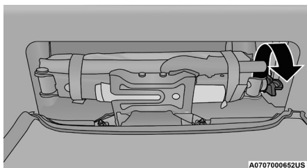
Retiro del gato
