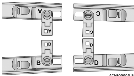
Posiciones de las barras transversales
