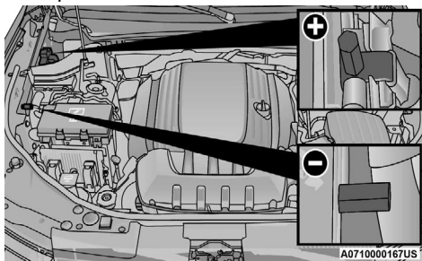
Terminales remotas de la batería
