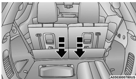
Desmontaje del piso alfombrado para tener acceso al anclaje de correa superior (3a. fila tipo banca)
