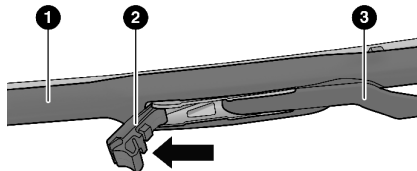
Pluma del limpiador con la pestaña en posición de liberación
