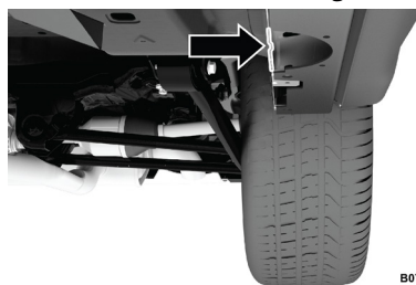
Punto de elevación trasero
