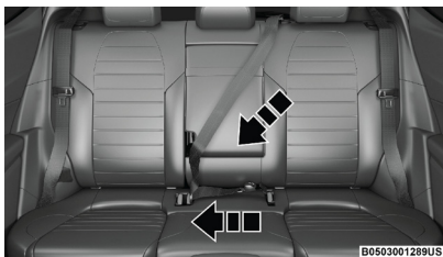
Insertando la contrahebillas a la hebilla
