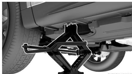
Ubicación frontal del gato
