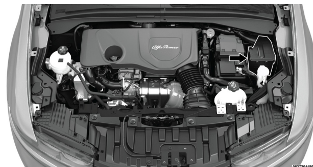
Ubicación del centro de distribución de energía — Motor 1.3L
