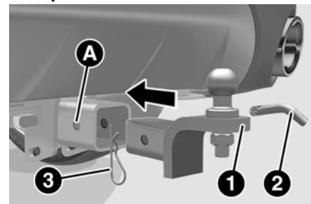
Ranura y receptor del remolque
