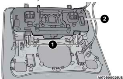
Compartimento de las luces de cortesía frontales
