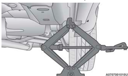
Ubicación para elevación con gato en la parte trasera
