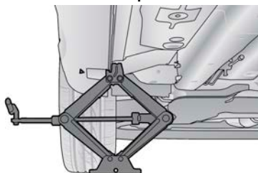
Ubicación para elevación con gato en la parte delantera
