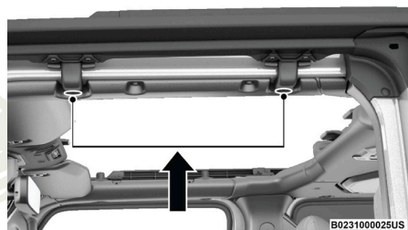
Ubicación de los tornillos del marco de la puerta
