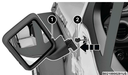
Conecte el mazo de cables al espejo exterior
