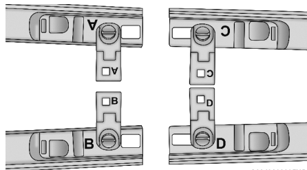
Posiciones de las barras transversales
