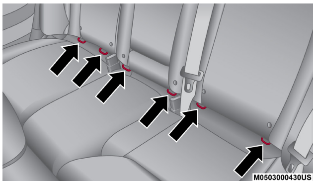
Anclajes LATCH
