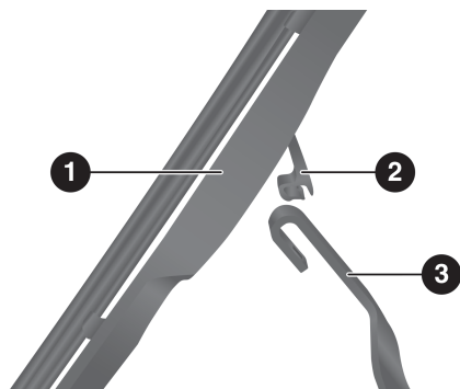
Desenganche del limpiador
