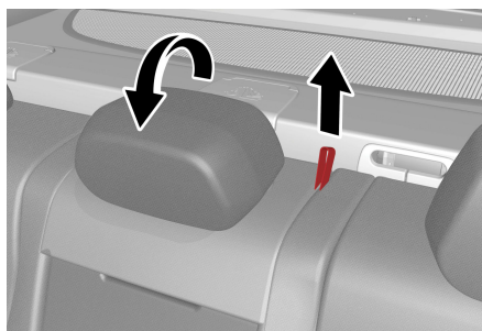
Abatimiento de la parte central del respaldo
