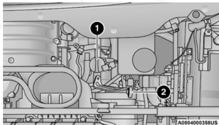
Ubicación de la varilla medidora y de llenado de aceite del motor
