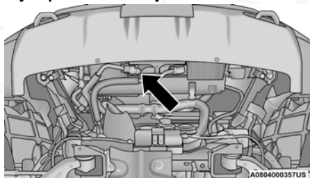
Drenaje del enfriador de aceite de motor
