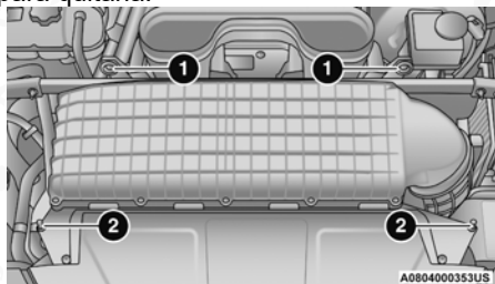
Puntos de sujeción de la cubierta de motor
