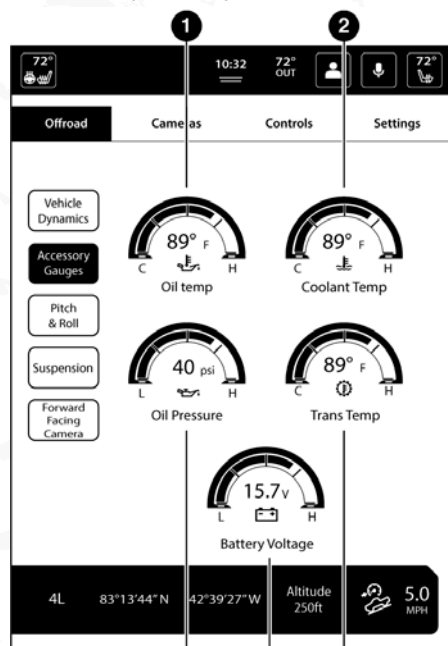
Menú del medidor de accesorios 2WD/4WD
