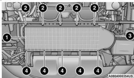
Filtro del aire acondicionado
