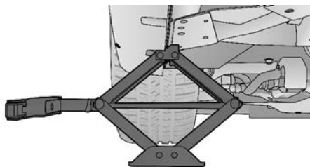
Ubicación delantera del gato
