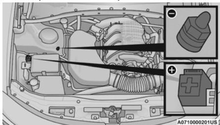
Localización de punto de arranque
