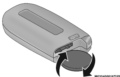
Separación de la cubierta usando una moneda
