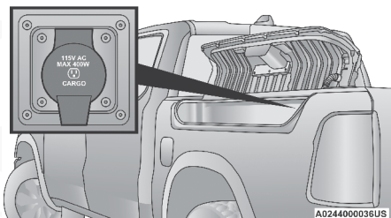
Inversor de corriente de la RamBox
