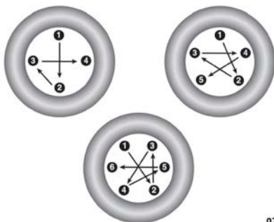
Patrón de apriete de 4, 5 y 6 tuercas
