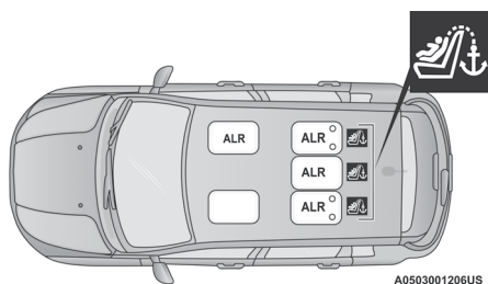
Ubicación de retractoros de bloqueo automático
