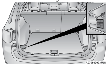
Ubicación de la caja de fusibles trasera
