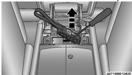
Liberación de la bisagra
