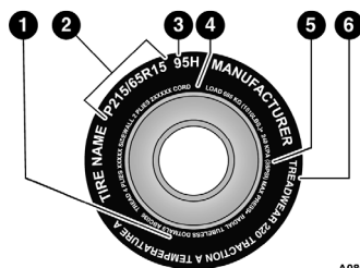
Marcado de la llanta
