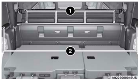
Retirar los fijadores Torx
