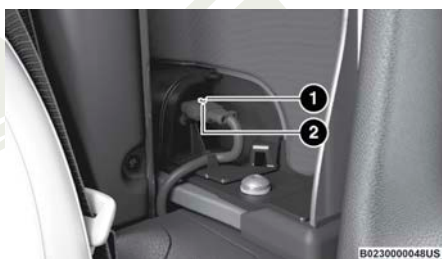
Liberación del arnés
