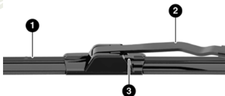
Pluma del limpiador con la pestaña en posición de bloqueo
