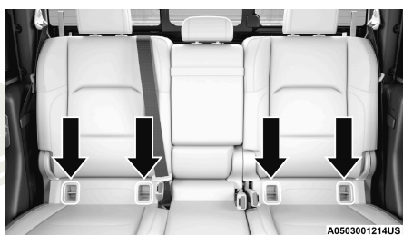
Anclajes LATCH
