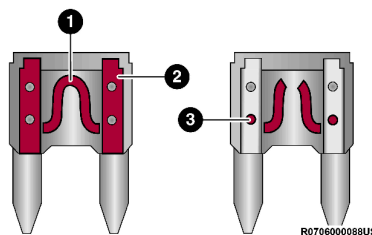
Hoja del fusible
