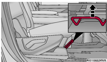
Palanca de ajuste del asiento trasero
