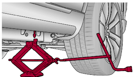
Ubicación trasera del gato
