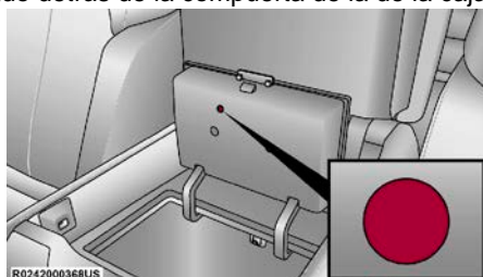
Ubicación del botón de restablecimiento
