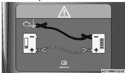
Etiqueta de conexión de cables pasacorriente
