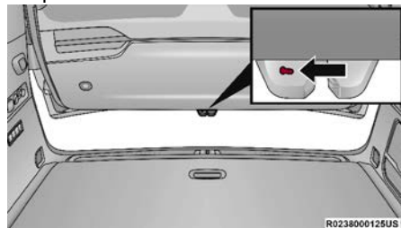
Liberación de servicio de la compuerta levadiza
