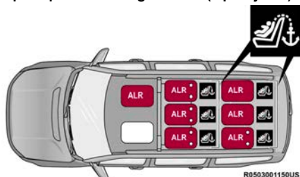
Ubicaciones del retractor de bloqueo automático (ALR) del banco de la segunda fila (8 pasajeros)
