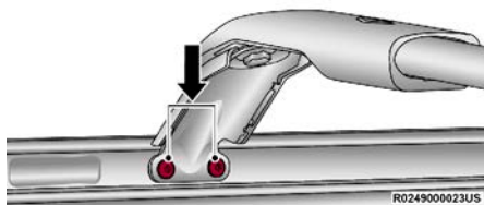
Ubicación de los tornillos
