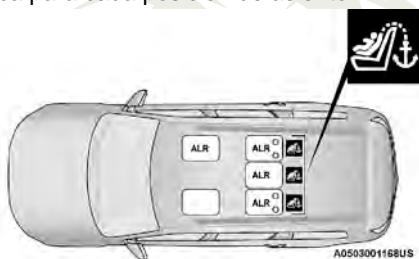
Ubicación de retractores de bloqueo automático (ALR) en vehículos de 5 asientos
