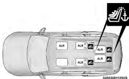
Ubicaciones ALR en vehículos de 6 pasajeros
