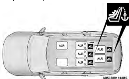
Ubicaciones ALR en vehículos de 7 pasajeros
