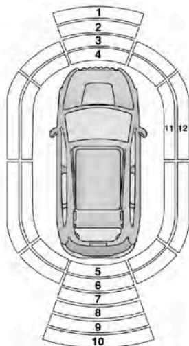
Arcos del ParkSense frontal/trasero
