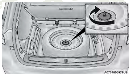
Reinstalación del sujetador de la llanta
