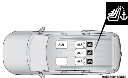
Ubicaciones ALR en vehículos de 5 pasajeros
