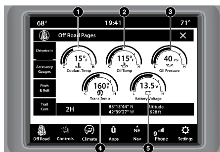
Menú de medidores de accesorios
