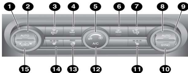
Sistema de control de clima automático (controles en el tablero)
