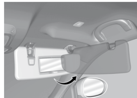
Rotación de la visera hacia la ventana del pasajero
