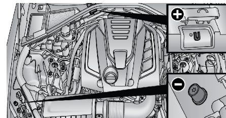
Ubicación de los postes remotos de la batería
