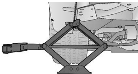
Ubicación delantera del gato
