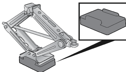
Uso del bloque de elevación de gato
