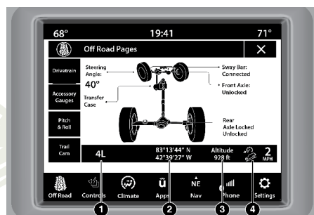
Barra de estado 2WD/4WD
