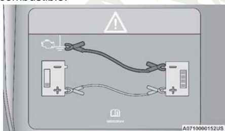
Etiqueta de inicio de conexión de cables pasa corriente
