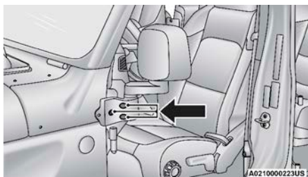
Ubicación de los tornillos del espejo
