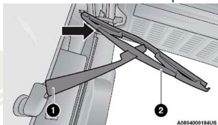
Hoja y brazo del limpiador
