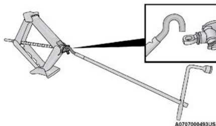
Gato ensamblado y herramientas
