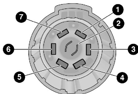
Conector de siete vías
