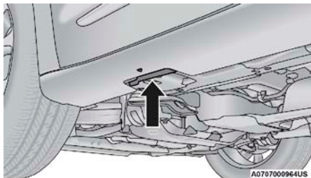
Ubicación delantera del gato
