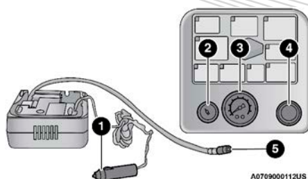
Compresor de aire portátil
