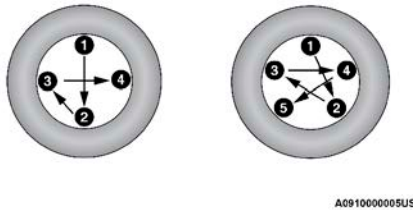
Patrón de apriete
