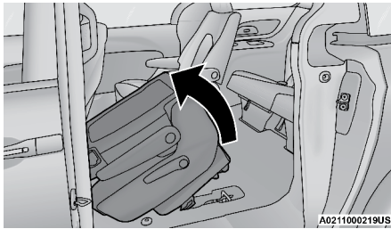
Inclinar el asiento hacia adelante
