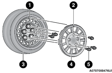
Cubiertas o tapas centrales de la llanta y rueda
