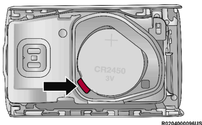
Apertura de retiro de batería
