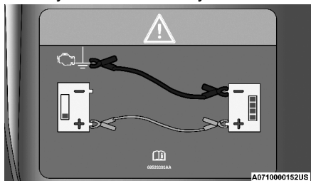
Etiqueta de conexión de cables puente
