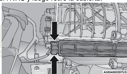
Lengüetas retenedoras del filtro de aire
