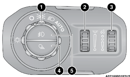
Interruptor de los faros de niebla
