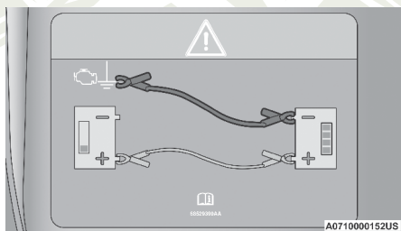
Conexiones de cables puente
