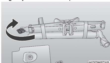
Tornillo de fijación del gato
