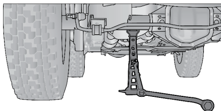
Punto de levantamiento en la parte trasera
