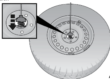
Reinstalando el retenedor
