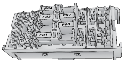
Panel de fusibles
