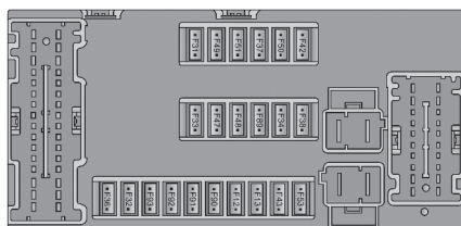
Ubicación de los fusibles del panel
